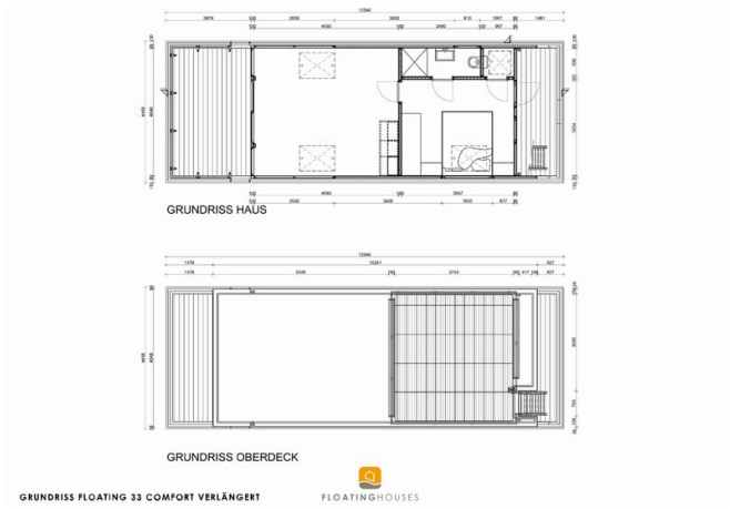
Grundriss_Hausboot_FH33_comfort_verlaengert
